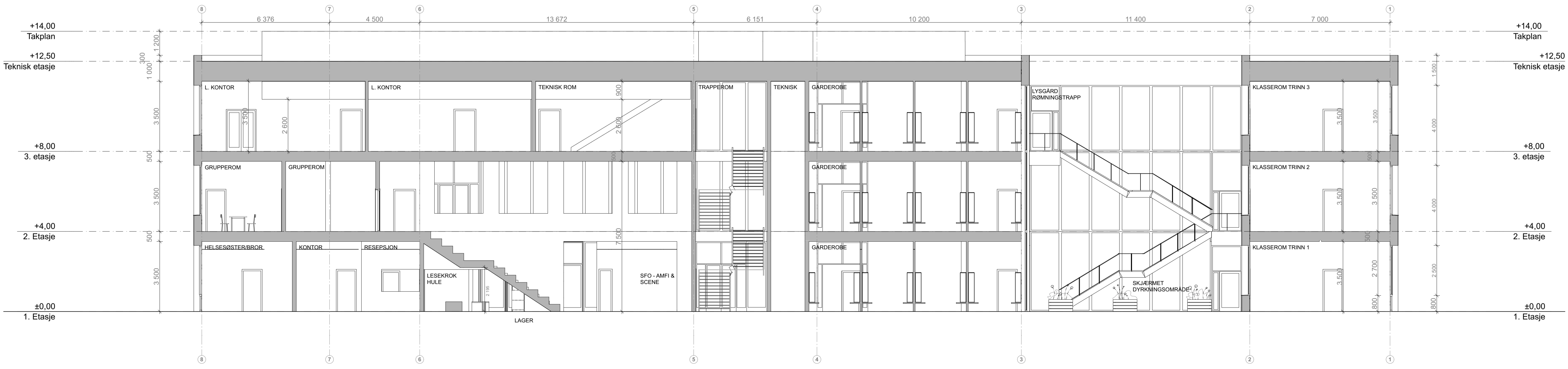
Snitt B 1:100
