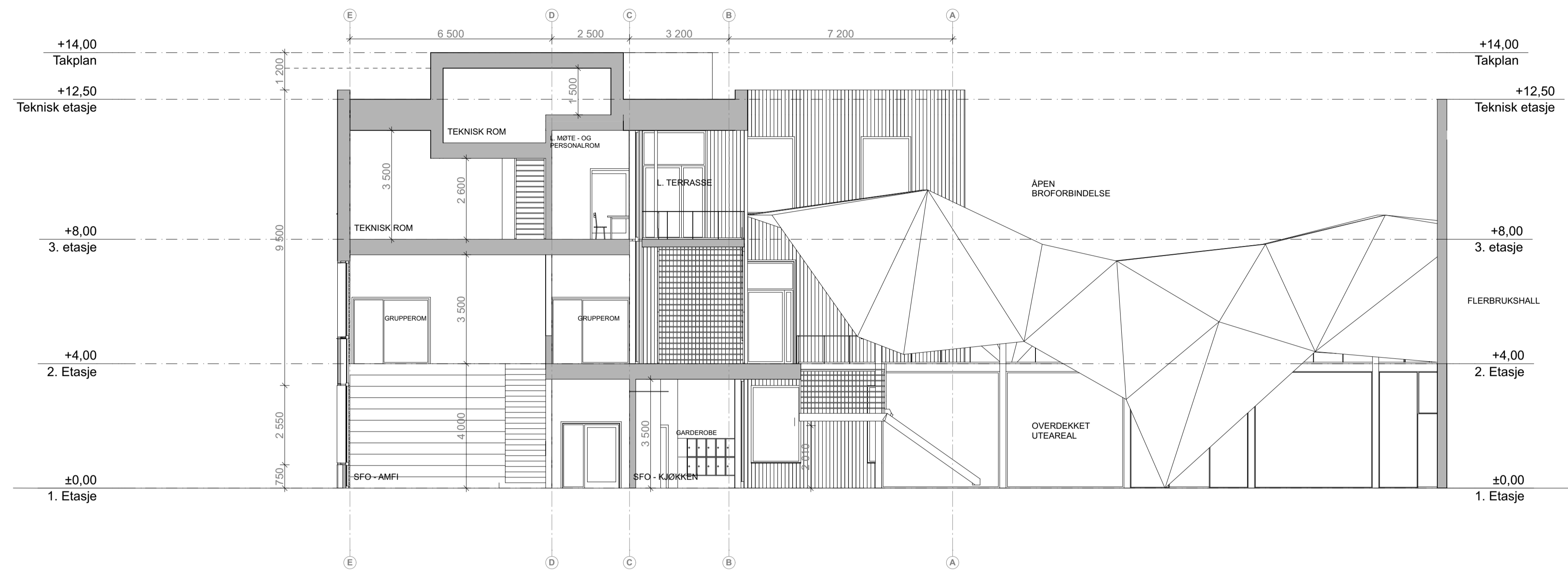
Snitt A 1:100
