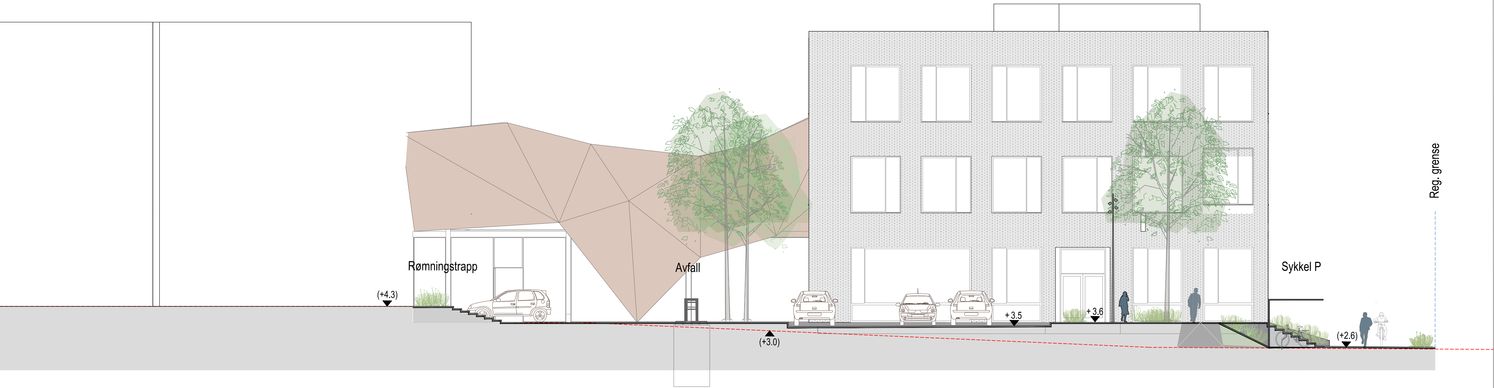
TERRENGSNITT B-B' PARKERINGSPLASS/ ADKOMSTTORGET
