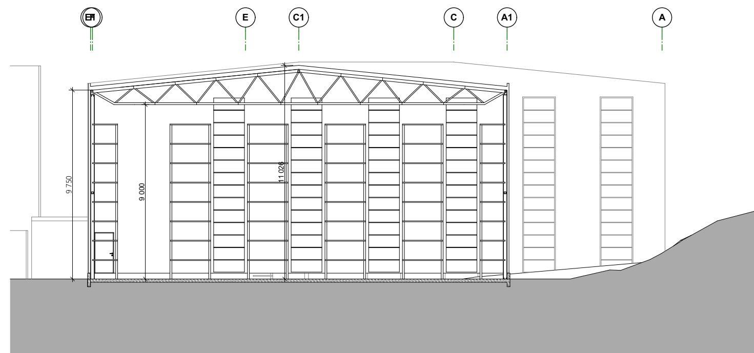
Snitt 12
