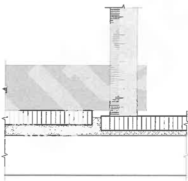
Fig. 51 d Måling av sprang ved fuger
