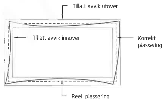
Fig. 61 Plassering i forhold til tillatt sammensatt byggtoleranse
