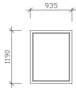
V-2 935x1190 ÅPNINGSBART Antall 8
