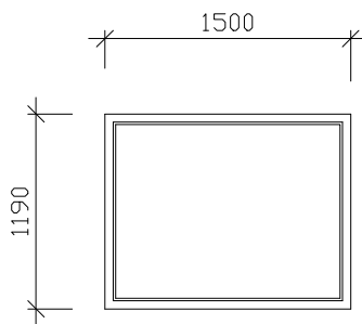
V-6 1500x1190 ÅPNINGSBART Antall 1
