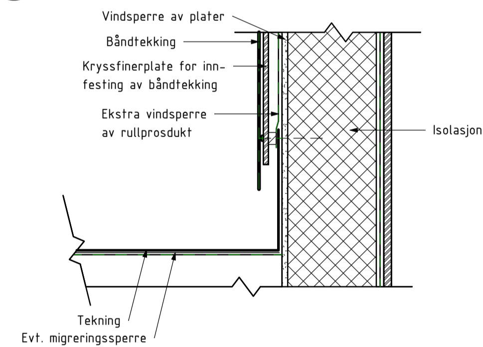
10 Detalj 10, oppbrett takpapp og beslag på "parapet" kulturskole G1 1 : 10
