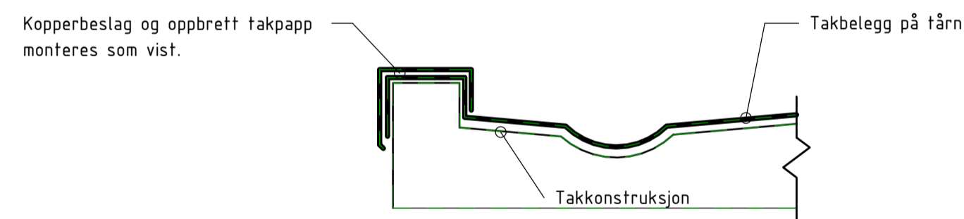
03 Detalj 03, Oppbrett gesimskant tårn 1 : 10
