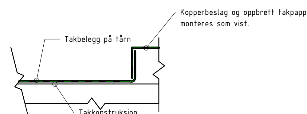
04 Detalj 04, Tårntak, oppbrett under beslag på sokkel 1 : 10
