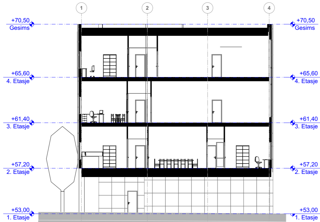
Snitt B
