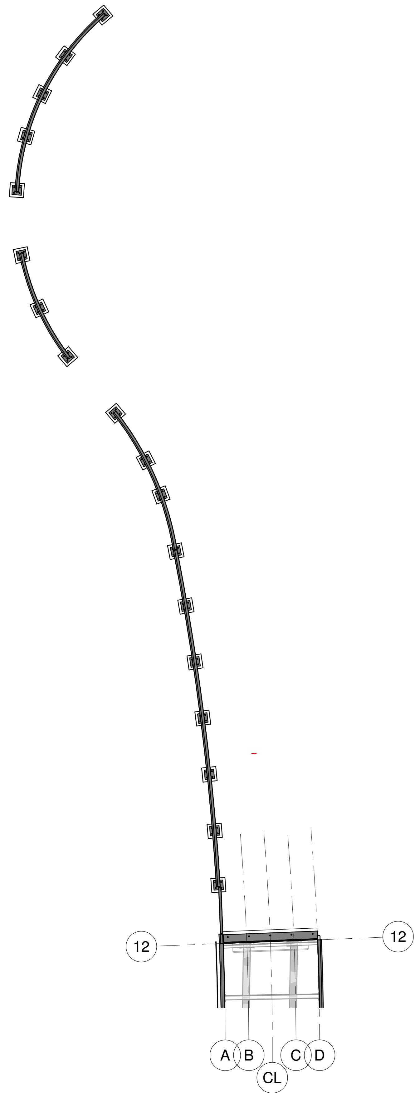
Plan nordside bro 1 : 50
