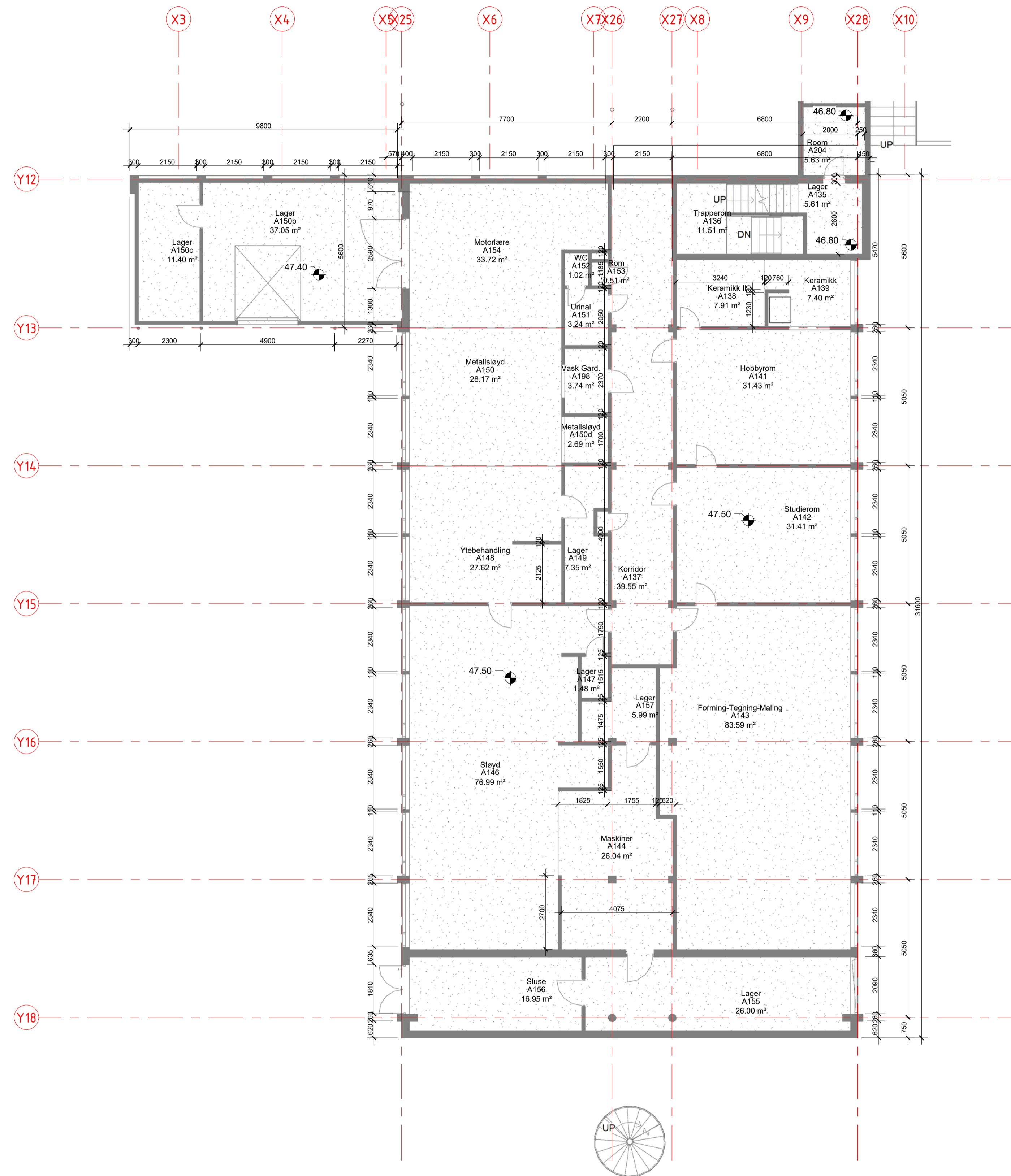
Plan Fløy A (kote 47.5) 1 : 100
