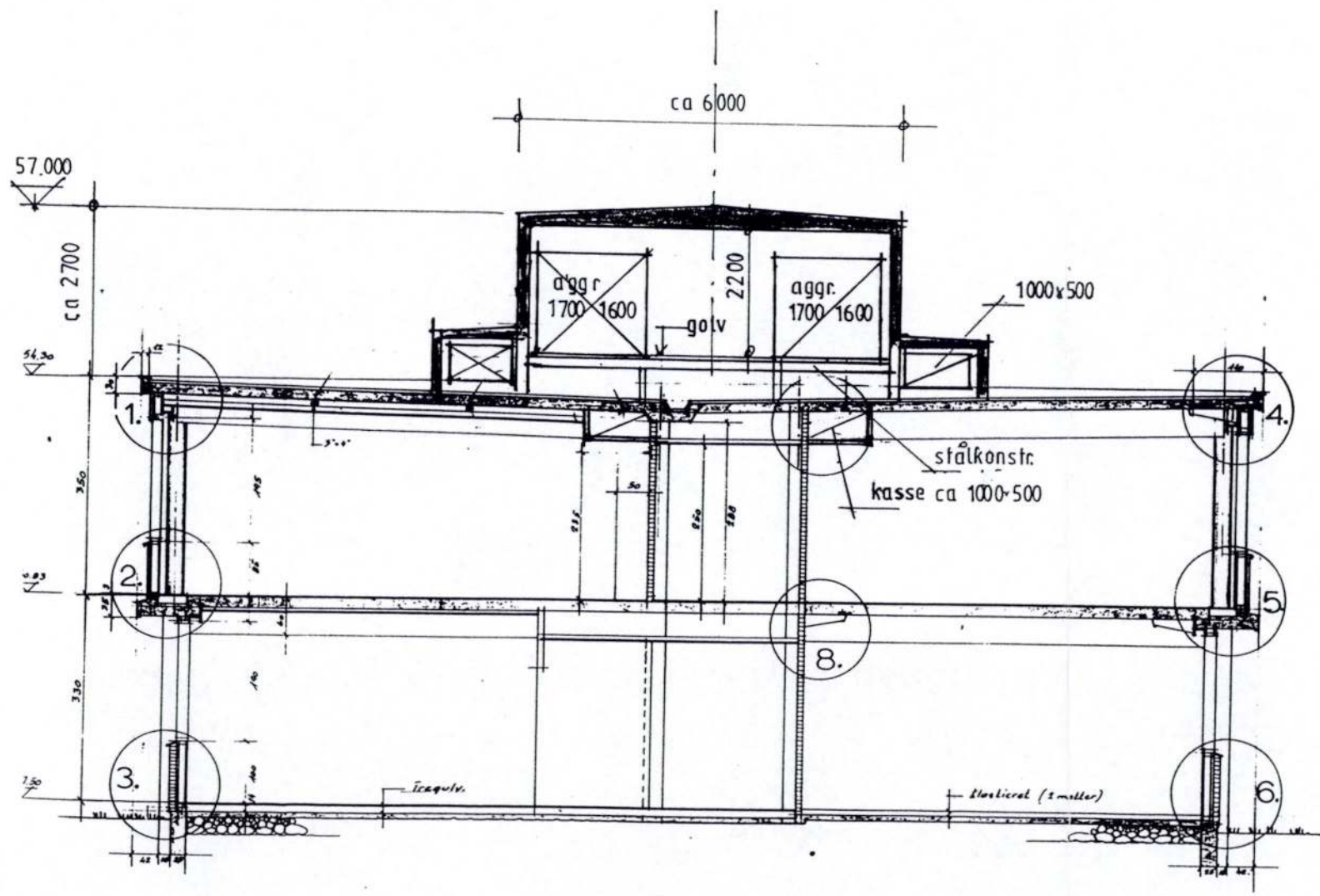
SNITT A-A
