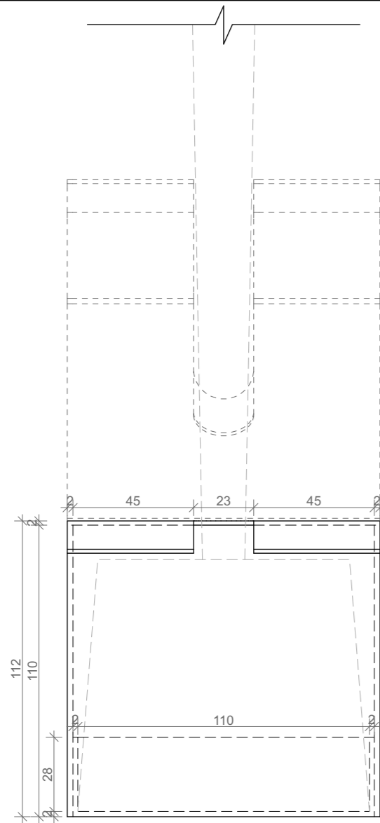
OPPRISS A-A
