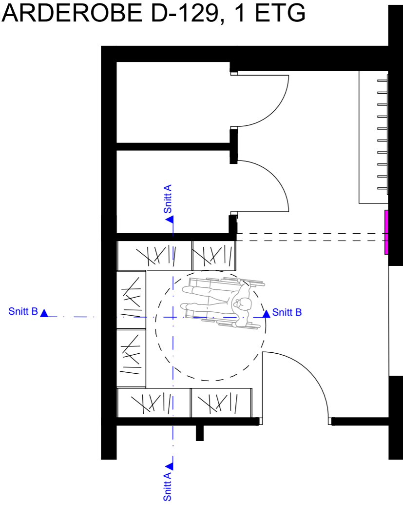
Plan 1:50
