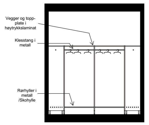
Snitt A-A 1:50
