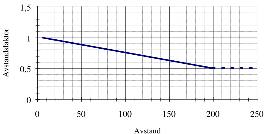
Figur. Avstandsfaktor som funksjon av korteste avstand mellom sprengningsstedet og de berørte bygg eller konstruksjoner.
