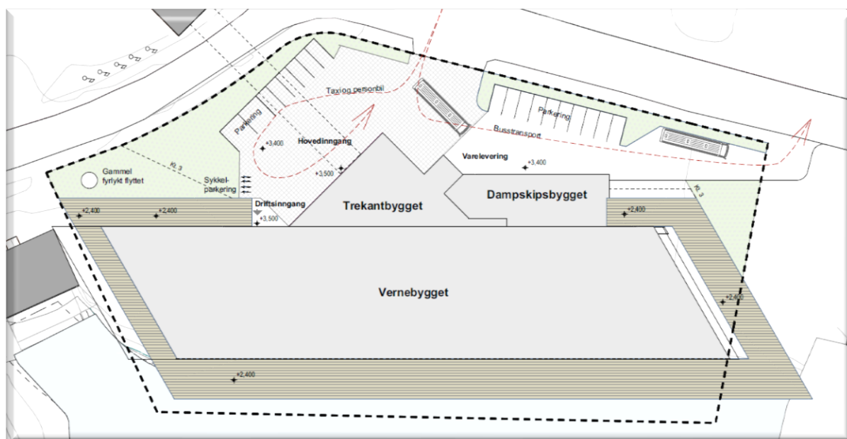
Figur 1: Situasjonsplan for vernebygg for M/S Finnmarken og nytt Hurtigrutemuseum
